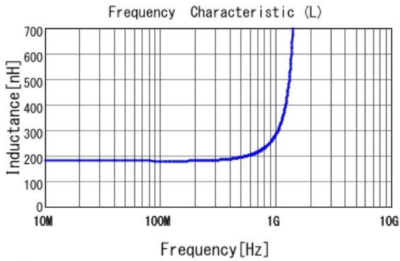
■ LQW18ANR18G00 L
