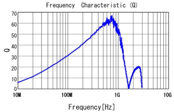
■ LQW18ANR18G00 Q
