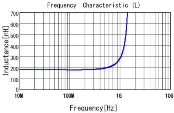
■ LQW18ANR18J00 L
