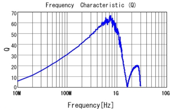
■ LQW18ANR18J00 Q
