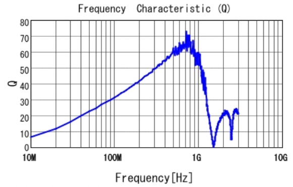
■ LQW18ANR22J00 Q
