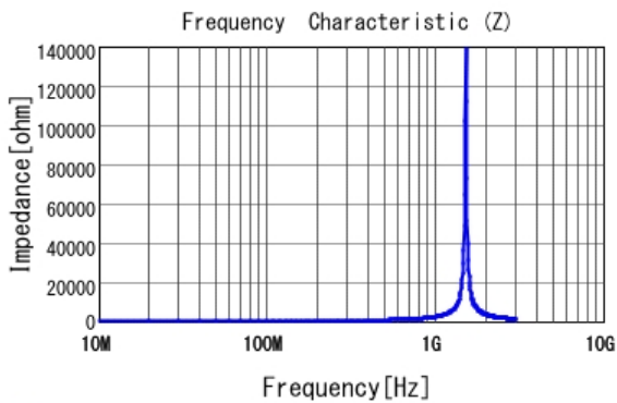
■ LQW18ANR22J00 |Z|
