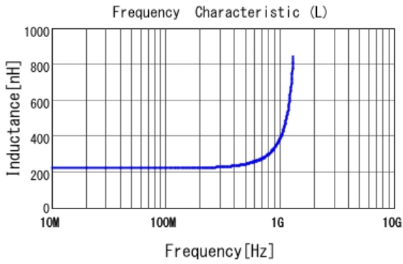
■ LQW18ANR22J00 L
