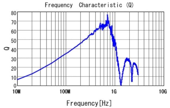
■ LQW18ANR27G00 Q
