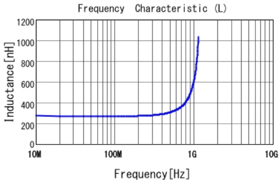
■ LQW18ANR27G00 L
