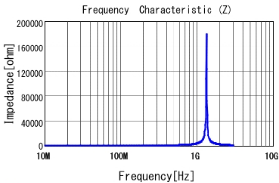
■ LQW18ANR27G00 |Z|
