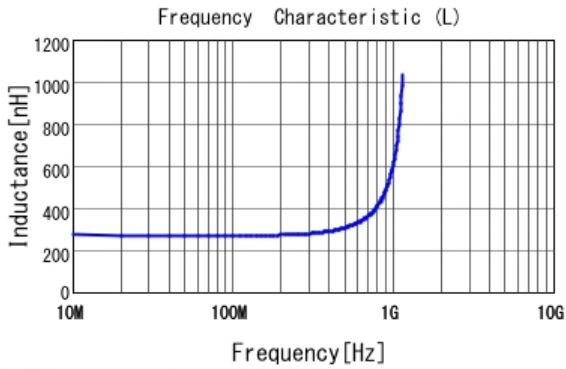
■ LQW18ANR27J00 L
