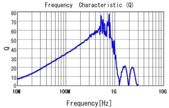
■ LQW18ANR30J80 Q
