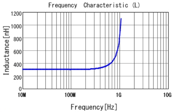
■ LQW18ANR30J80 L
