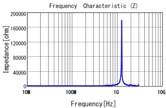
■ LQW18ANR30J80 |Z|
