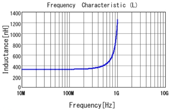
■ LQW18ANR33G00 L
