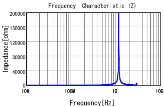
■ LQW18ANR33G00 |Z|
