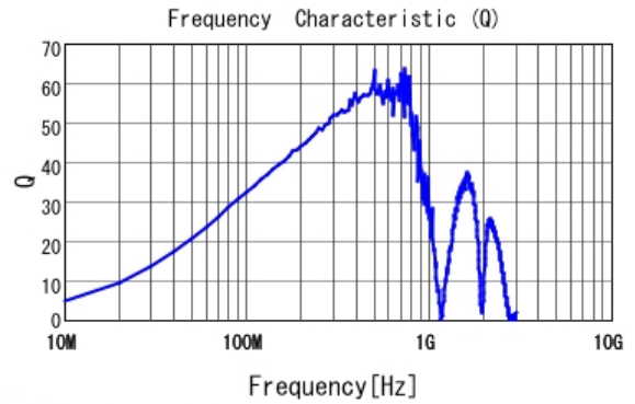
■ LQW18ANR33J00 Q
