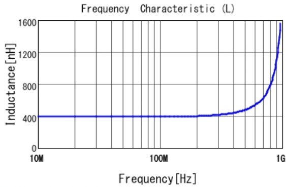
■ LQW18ANR39G00 L
