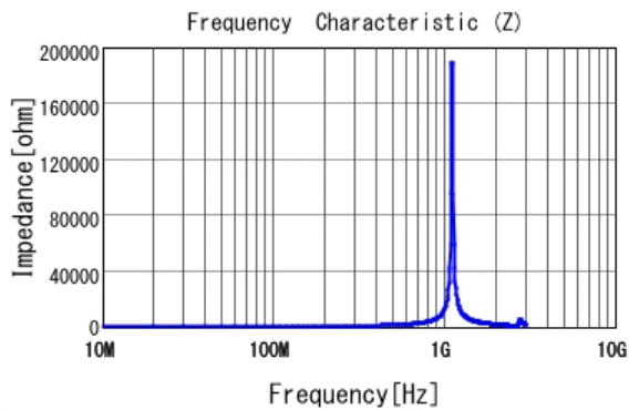
■ LQW18ANR39G00 |Z|
