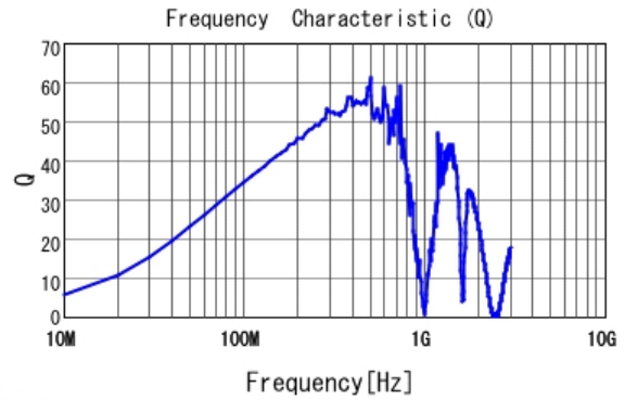
■ LQW18ANR47G00 Q
