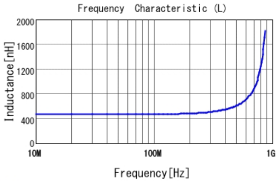
■ LQW18ANR47G00 L
