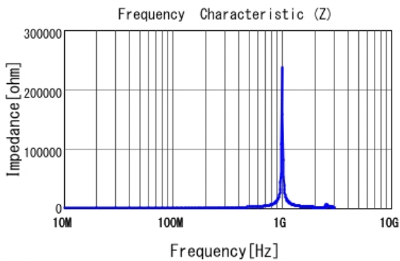
■ LQW18ANR47G00 |Z|
