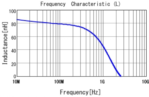
■ LQW18CN85NJ00 L
