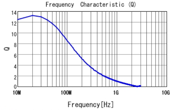
■ LQW18CN85NJ00 Q
