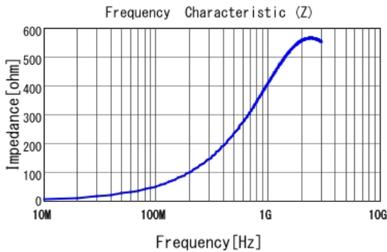
■ LQW18CN85NJ00 |Z|
