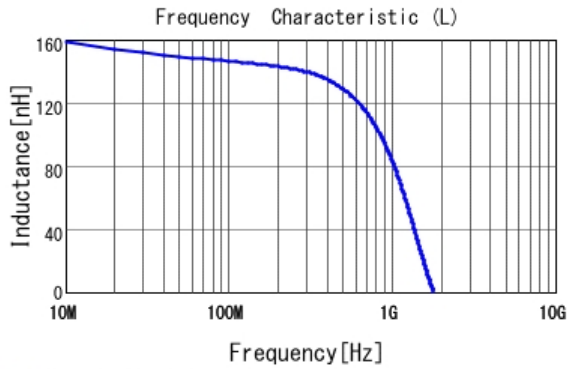
■ LQW18CNR16J00 L
