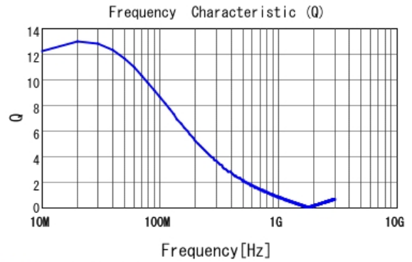
■ LQW18CNR16J00 Q
