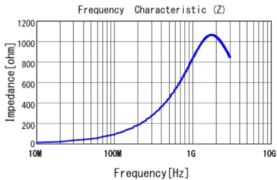
■ LQW18CNR16J00 |Z|
