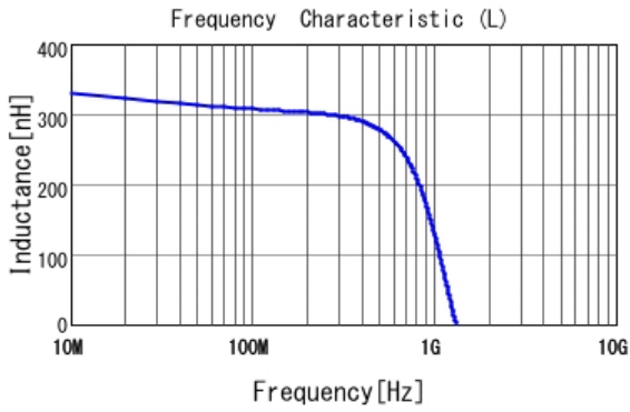
■ LQW18CNR33J00 L
