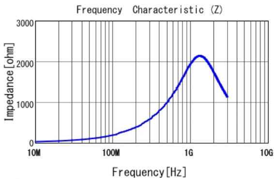
■ LQW18CNR33J00 |Z|
