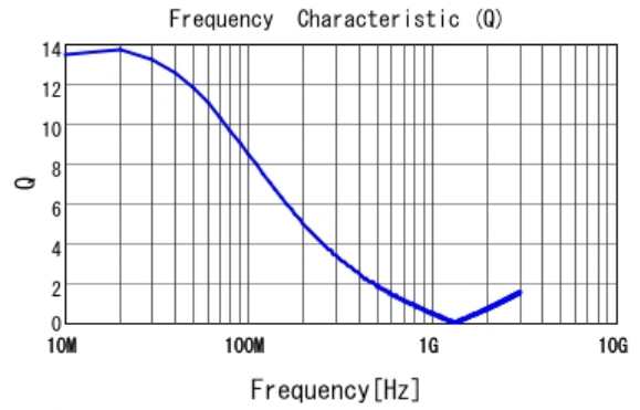
■ LQW18CNR33J00 Q
