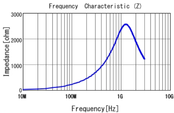
■ LQW18CNR39J00 |Z|
