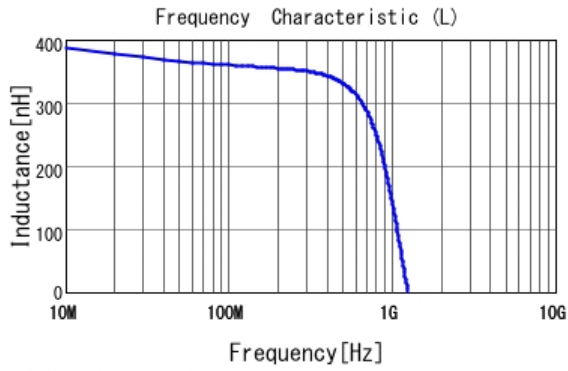
■ LQW18CNR39J00 L
