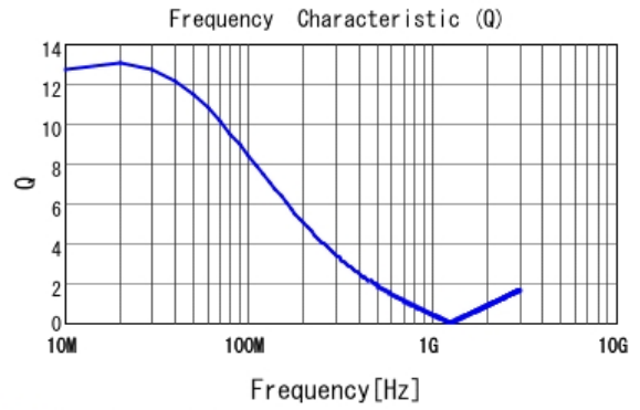
■ LQW18CNR39J00 Q
