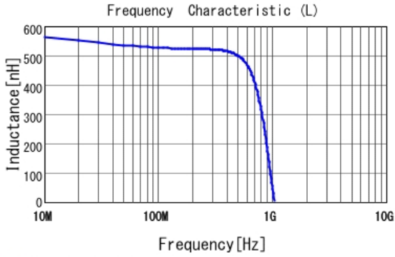
■ LQW18CNR56J00 L
