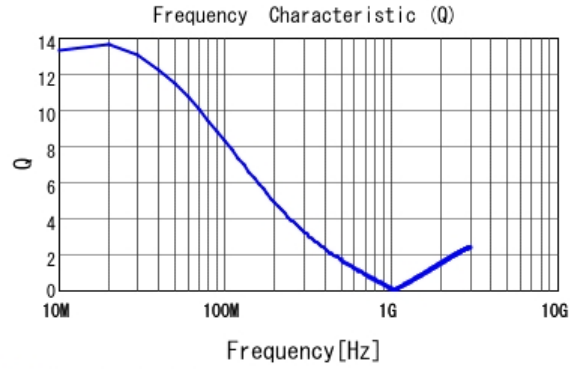
■ LQW18CNR56J00 Q
