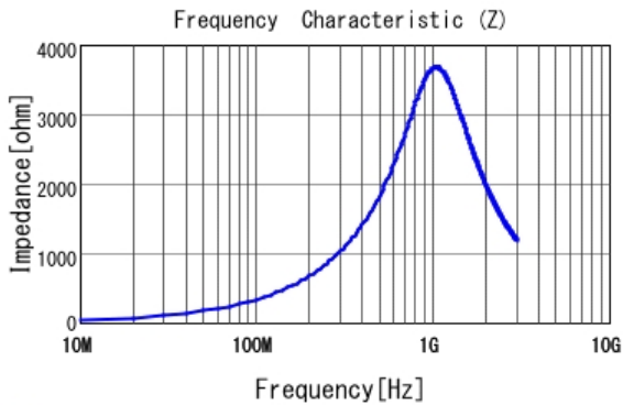
■ LQW18CNR56J00 |Z|
