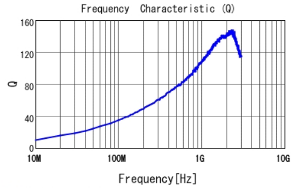
■ LQW2BAS10NG00 Q
