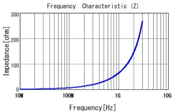
■ LQW2BAS10NG00 |Z|
