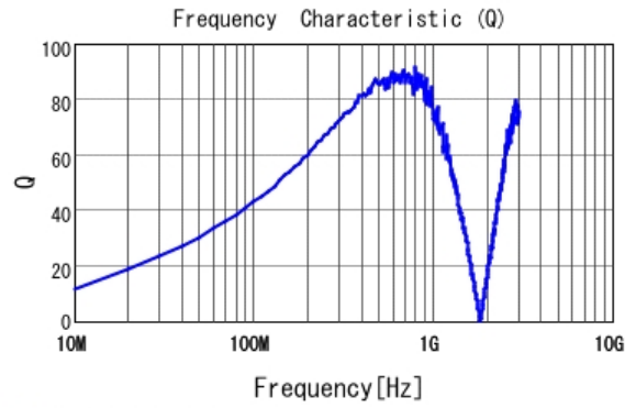
■ LQW2BAS68NJ00 Q
