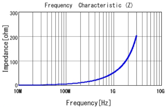
■ LQW2BAS8N2J00 |Z|
