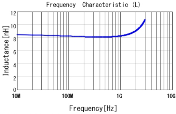
■ LQW2BAS8N2J00 L
