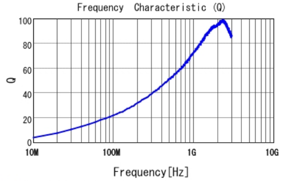
■ LQW2BAS8N2J00 Q
