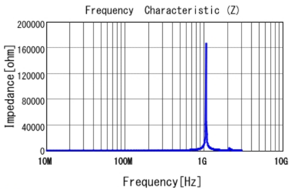
■ LQW2BASR18J00 |Z|
