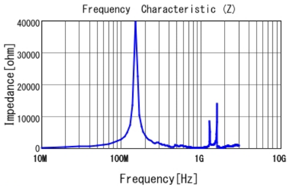
■ LQW2UAS2R7J00 |Z|
