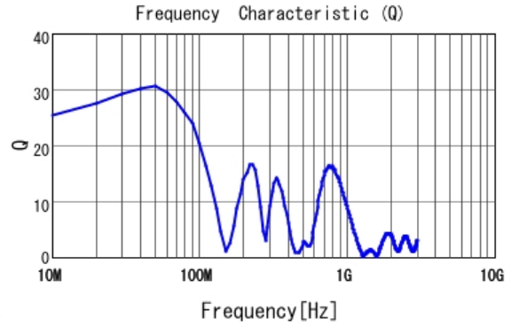
■ LQW2UAS2R7J00 Q
