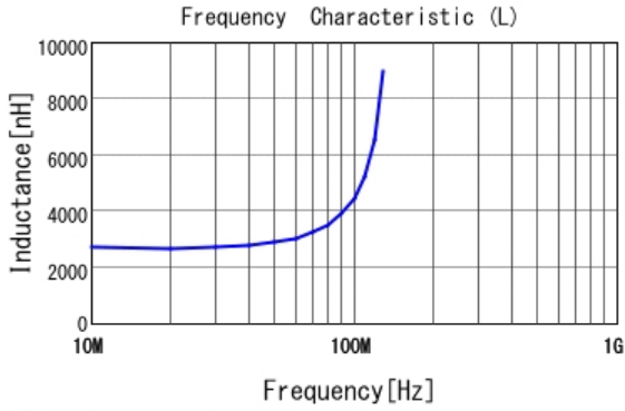
■ LQW2UAS2R7J00 L
