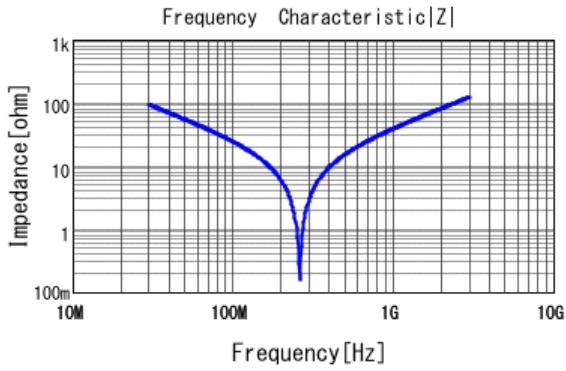
■ RCE5C1H560J0K1H03B |Z| DCOV, 25degC
