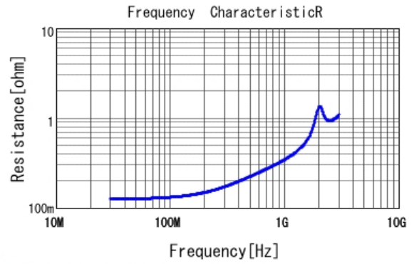
■ RCE5C1H560J0K1H03B R DCOV, 25degC
