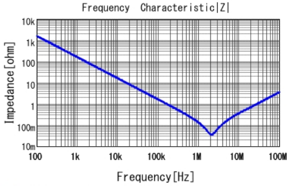
■ RCER71H105K2K1H03B |Z| DCOV, 25degC
