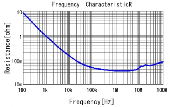
■ RCER71H105K2K1H03B R DCOV, 25degC
