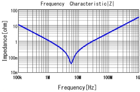
■ RCER71H154K1K1H03B |Z| DC0V, 25degC
