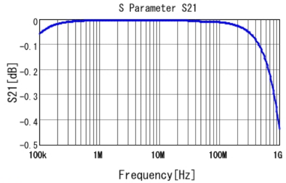
■ RCER71H154K1K1H03B S21 DC0V, 25degC
