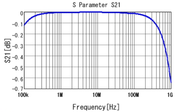
■ RDER71H104K0K1H03B S21 DC0V, 25degC
