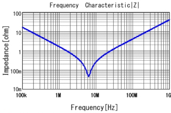
■ RDER71H104K0K1H03B |Z| DC0V, 25degC
