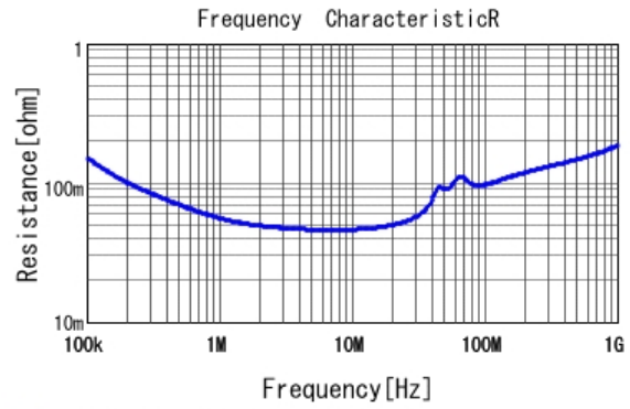
■ RDER71H104K0K1H03B R DC0V, 25degC
