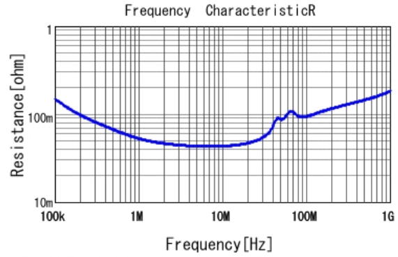
■ RDER71H104K0S1H03A R DC0V, 25degC
