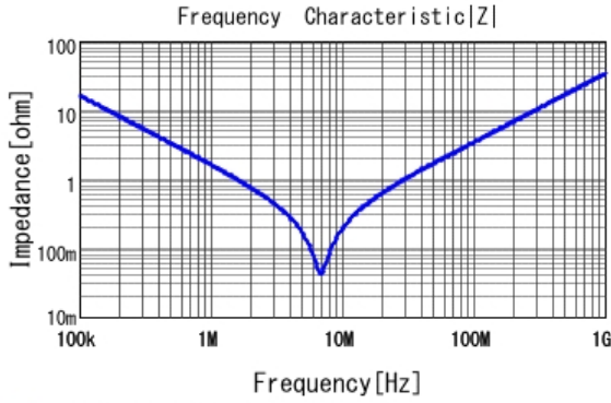
■ RDER71H104K0S1H03A |Z| DC0V, 25degC
