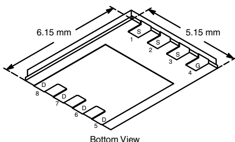
PowerPAK® SO-8
