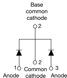
VS-43CTQ...-1-M3
